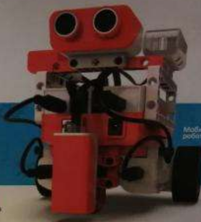
Ультразвуковой датчик
